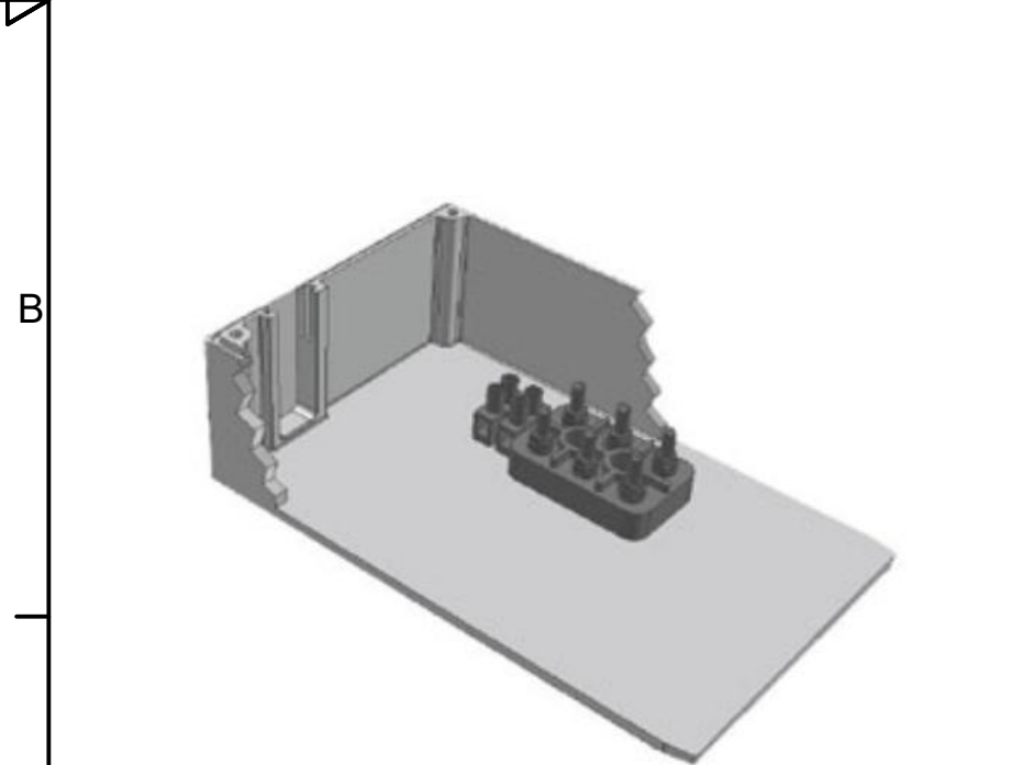
Klemmenkasten (Endschaltergehäuse ohne Schaltmechanik).
